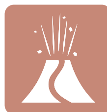
Super-volcano
